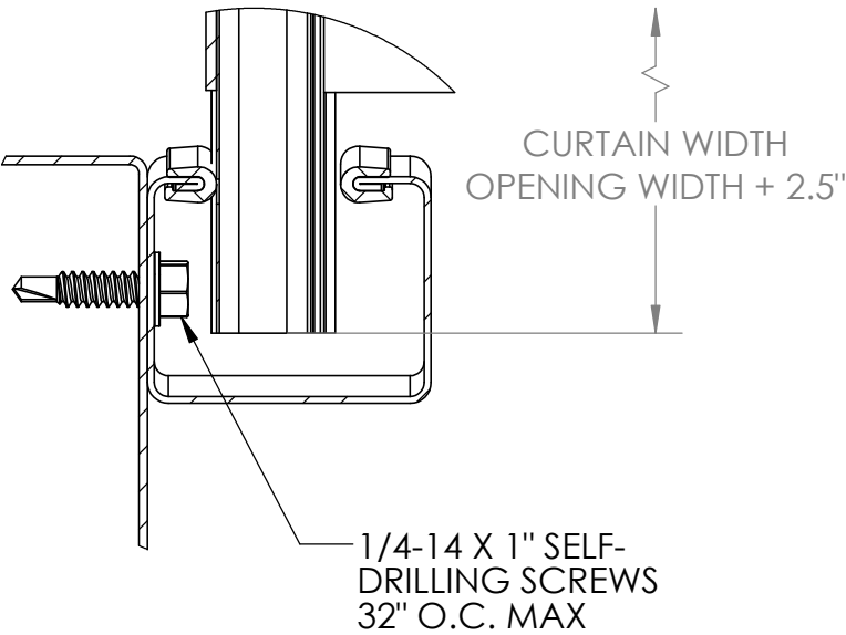
DOOR GUIDE TO STEEL JAMB
