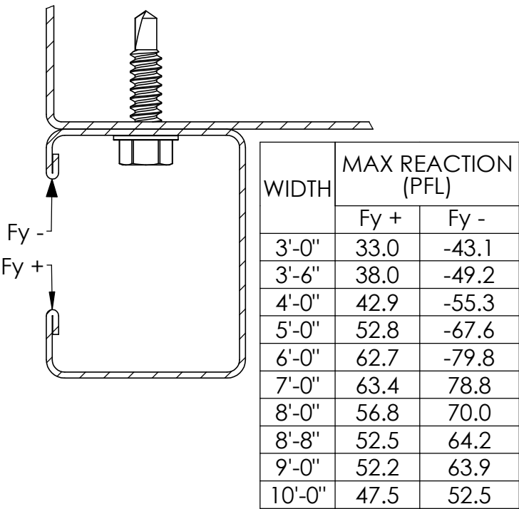
DOOR GUIDE FORCE
